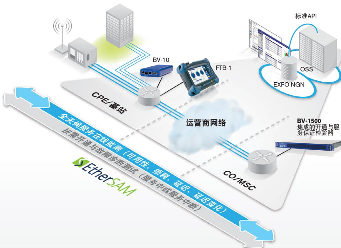
图1: BV-1500是EXFO的Ethernet One解决方案的组成部分，用于端到端以太网测试和监测。
