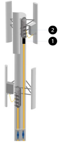
FTTAジャンクションボックスとRRUを接続するジャンパー
