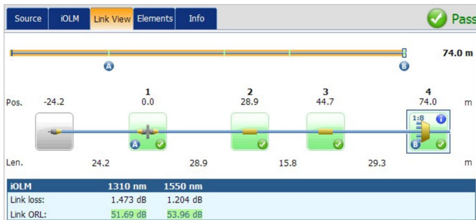
図3.テストパスラストマイル損失およびORLは仕様範囲内です。スプリッターの存在が確認され、予想比率と照合し、フィーダーへの継続性があります。ラストマイル敷設が保証されます。
