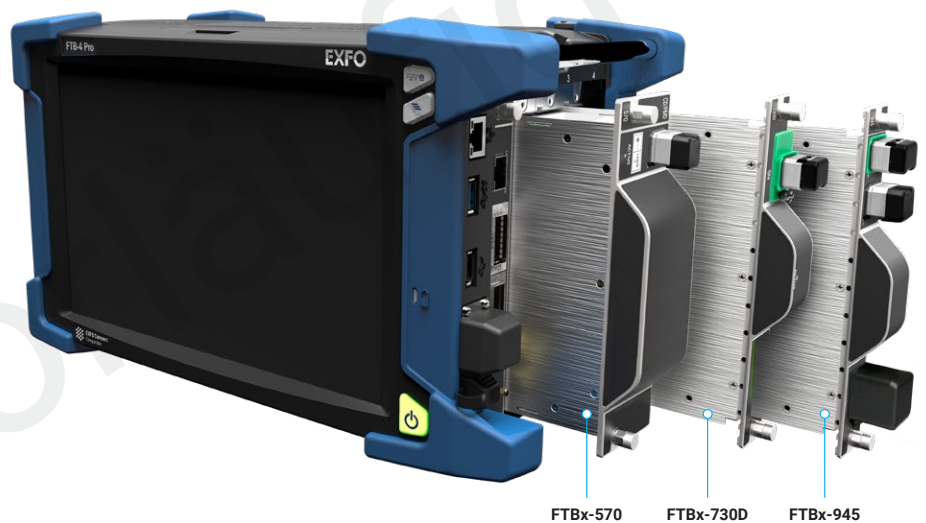
FTBx-570
