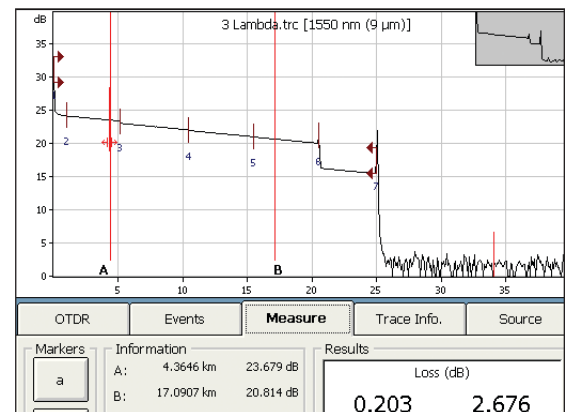
Mediciones de pérdidas desde la curva de OTDR de 1550 nm.
