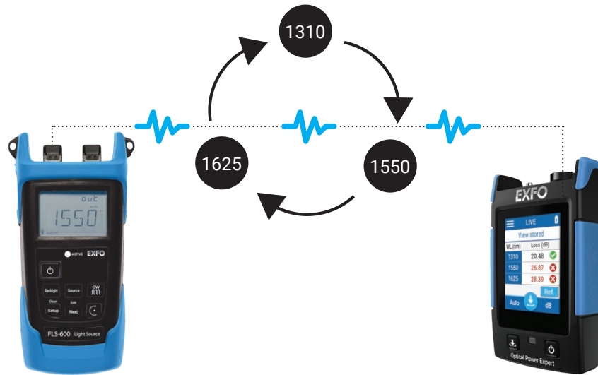
Commutation automatique de la vitesse de longueur d'onde Source optique
