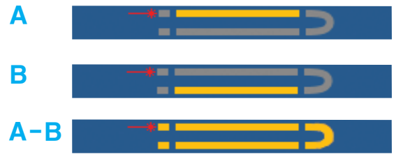
iOLM에서 루프백 테스트 방식과 iLOOP 옵션을 사용하면 피이버 두 개를 한꺼번에 테스트할 수 있습니다. A 링크만, B 링크만 보거나 루프까지 포함해 A-B 링크 전체를 볼 수 있습니다.
